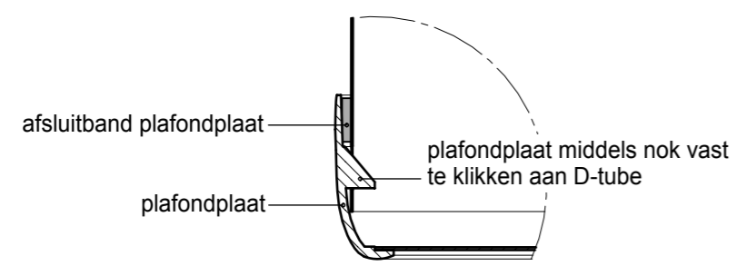
Detail aansluiting plafondplaat Schaal 1:2
