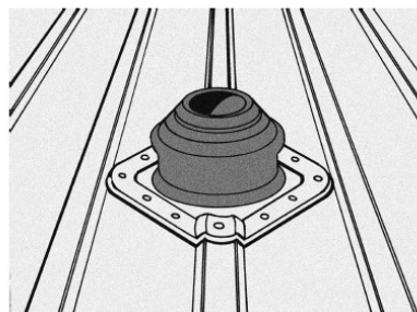
Plaats doorvoer diagonaal bij grote gaten en in geval van hoge profilering
