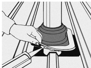
Breng aan onderzijde bevestigingsrand een neutrale siliconenkit aan
